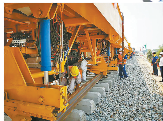
3月27日，中老铁路老挝段正式开始铺轨。中铁十五局集团路桥公司负责中老铁路老挝段全线801257根轨枕、259组道岔枕的生产。图为中老铁路正在铺设轨枕。 李红文 李永 摄
